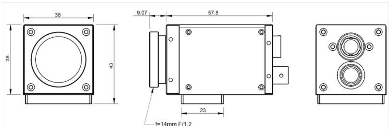
VIM-640G2N*カメラの外形図
