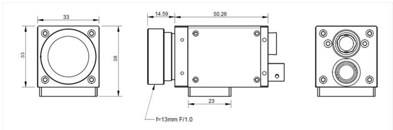
VIM-384G2N*カメラの外形図
